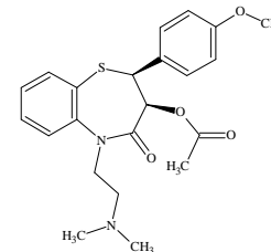
Diltiazem
